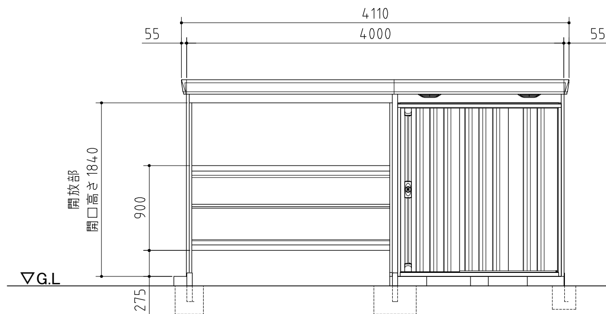
正面図
